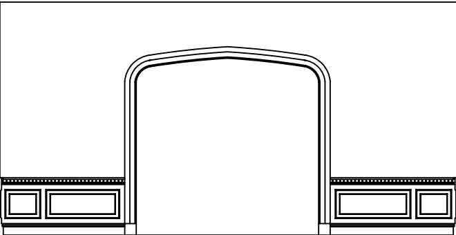
E1/A3.1 1/2" = 1'-0"
