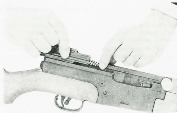
Fig. 15. — Remontage du couvre-culasse
