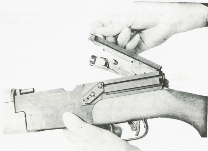
Fig. 14. — Démontage de l'ensemble mobile
