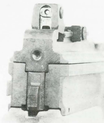
Fig. 6. — Œillette réglable du F.S.A. 1949-56 [vue arrière droit]
