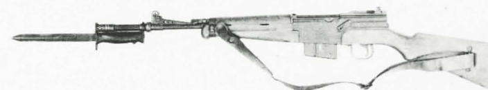
Fig. 1. — Fusil S.A. 1949-56 avec couteau-baïonnette et chargeur [vue latérale gauche]
