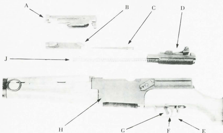
A. Pièce de manœuvre. B. Culasse. C. Percuteur. D. Couvre-culasse. E. Pontet.
