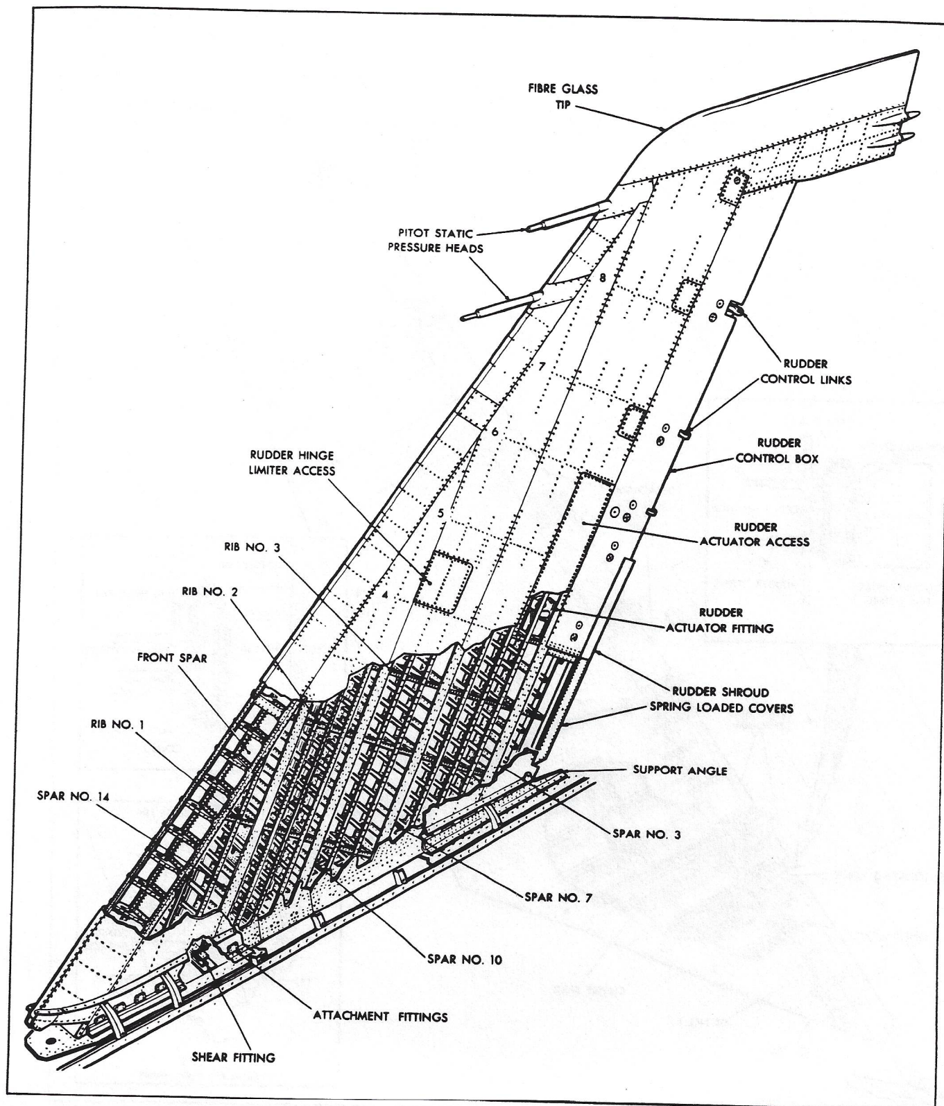
FIN STRUCTUE
