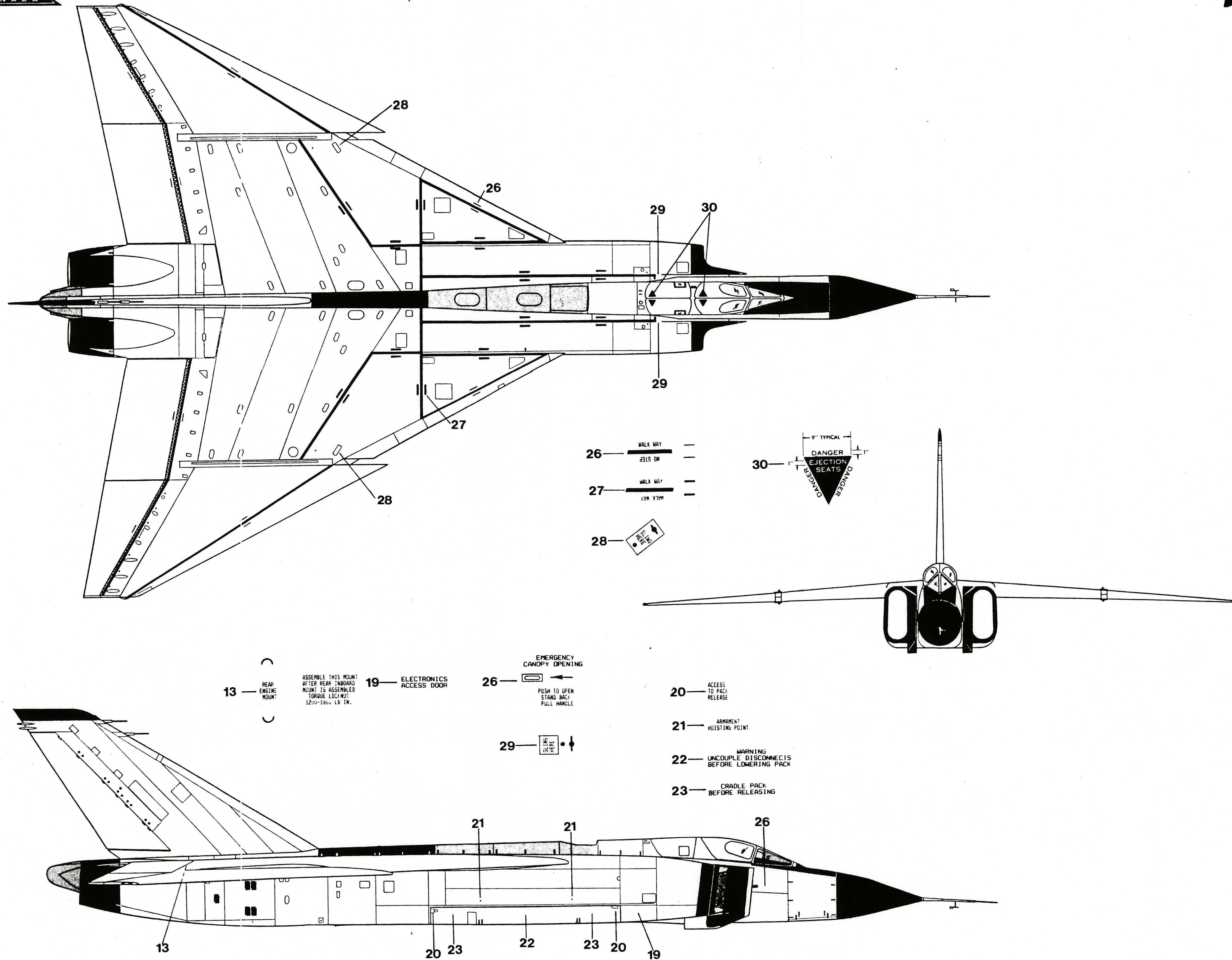
AVRO ARROW MK 1
