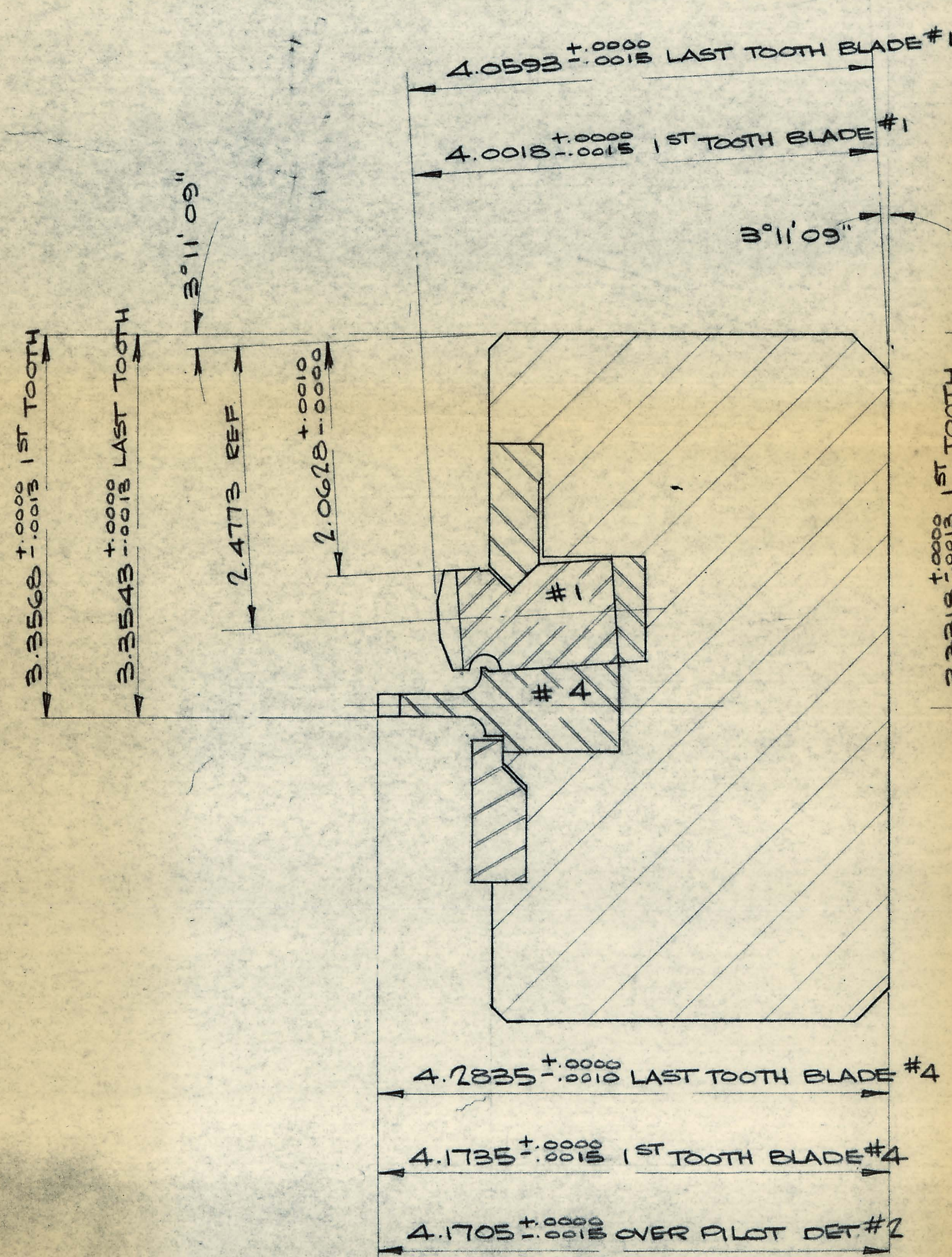
SECTION A-A
