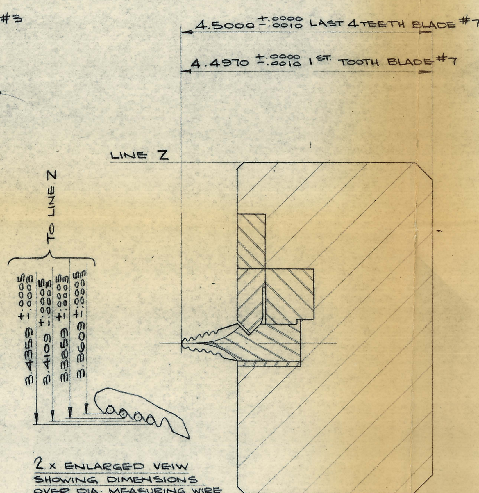
SECTION D-D
