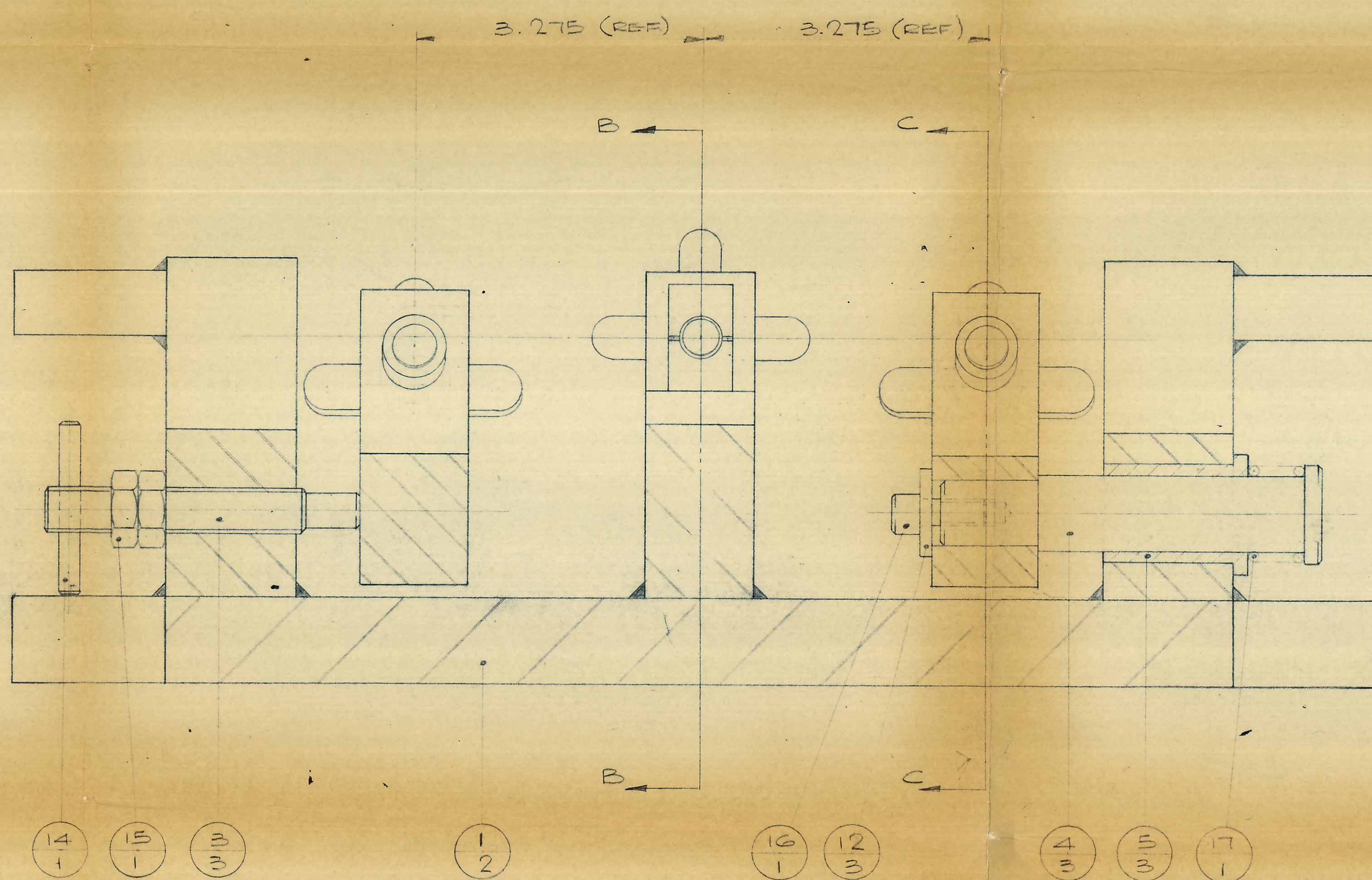
SECTION A-A
