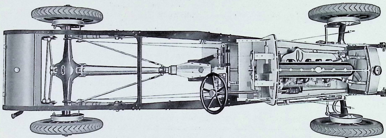
Châssis "Excelsior,, Type Albert I er . 6 cylindres, 35 CV, vu en plan.
