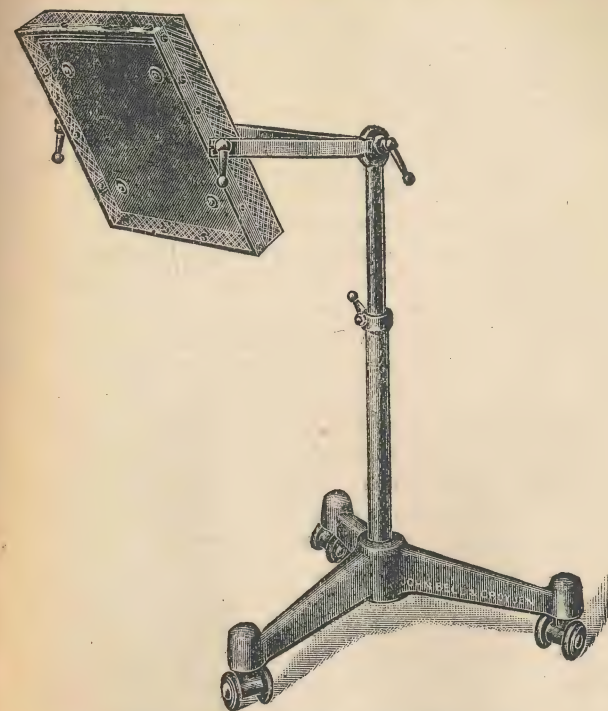
(FIG. 12.) "ARNOLD" INFRA-RED LAMP.
