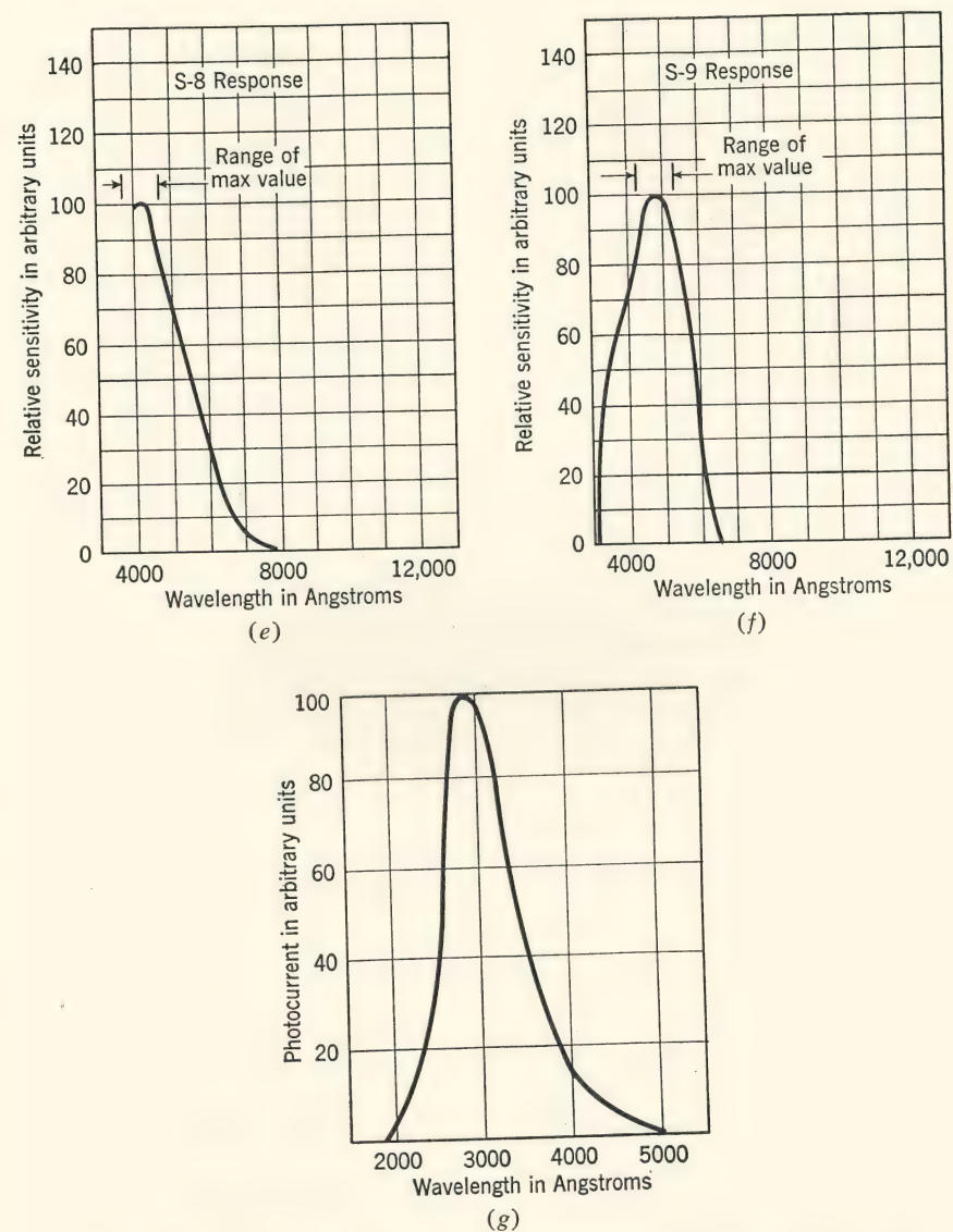
FIG. 8 (Continued). e and f. RCA Bulletin CRPS-102-A. g. S-6 sodium.
