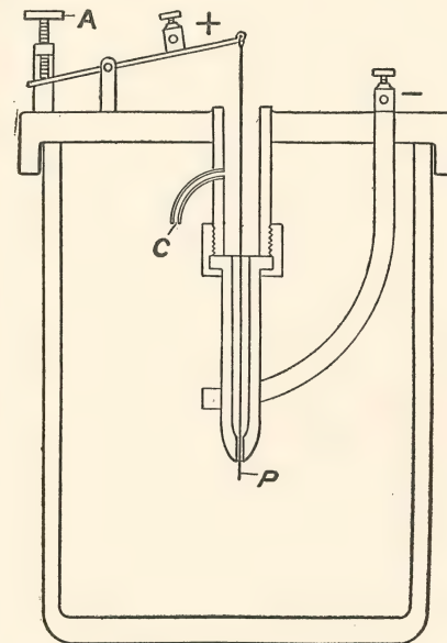
FIG. 10.—WEHNELT INTERRUPTER.
