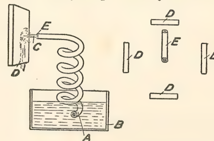
FIG. 7.—MERCURY-JET INTERRUPTER.
