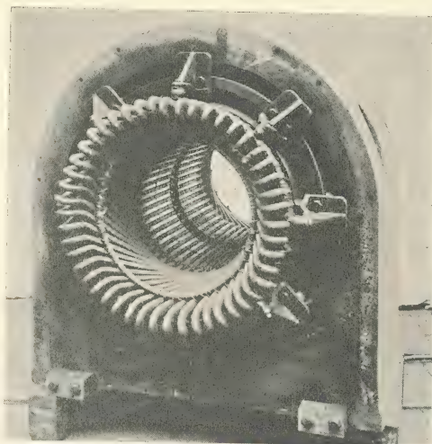
FIG. 29—STATOR OF 625 K.V.A., 2 300 VOLTS, 3 600 R. P. M., TURBO-GENERATOR
