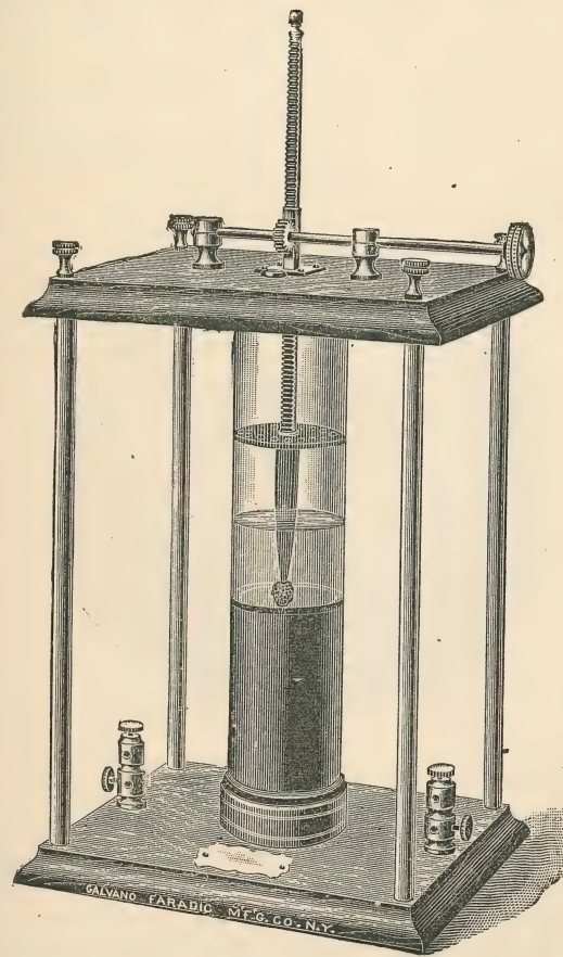
Rheostat.
