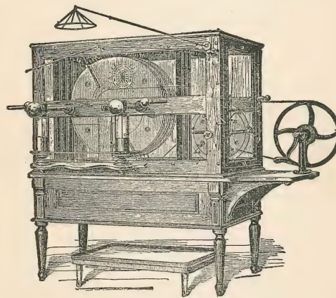
Static Machine (Waite & Bartlett.)
