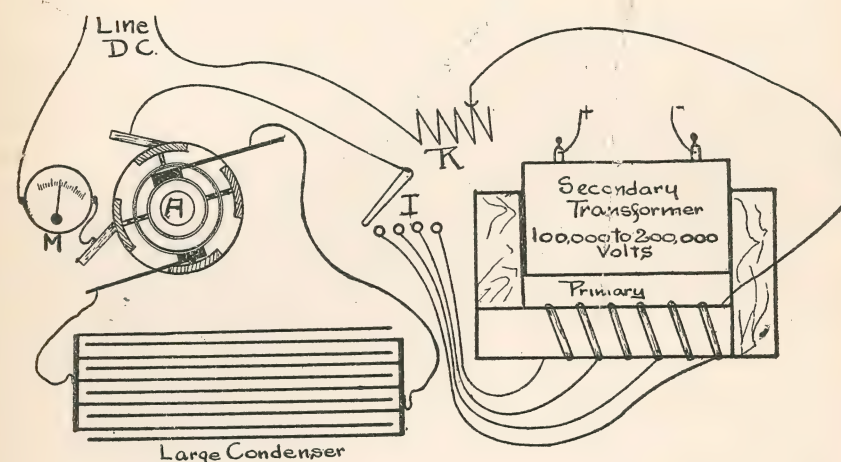
FIG. 27. McCaa Transformer.
