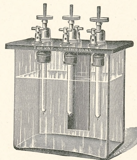
FIG. 74.—Wehnelt interrupter.
