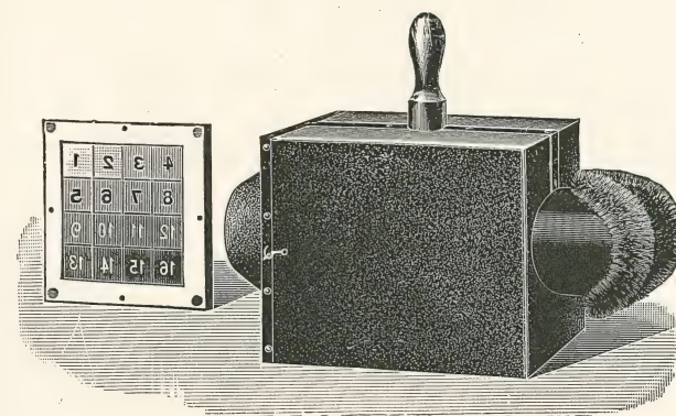
FIG. 219.—The skiameter.
