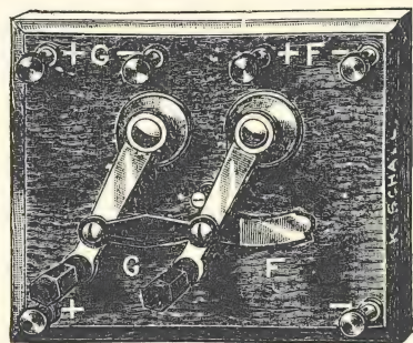
FIG. 48.—DE WATTEVILLE COMMUTATOR
