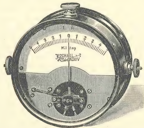
FIG. 24.—THE D'ARSONVAL MILLIAMPÈRE METER.
