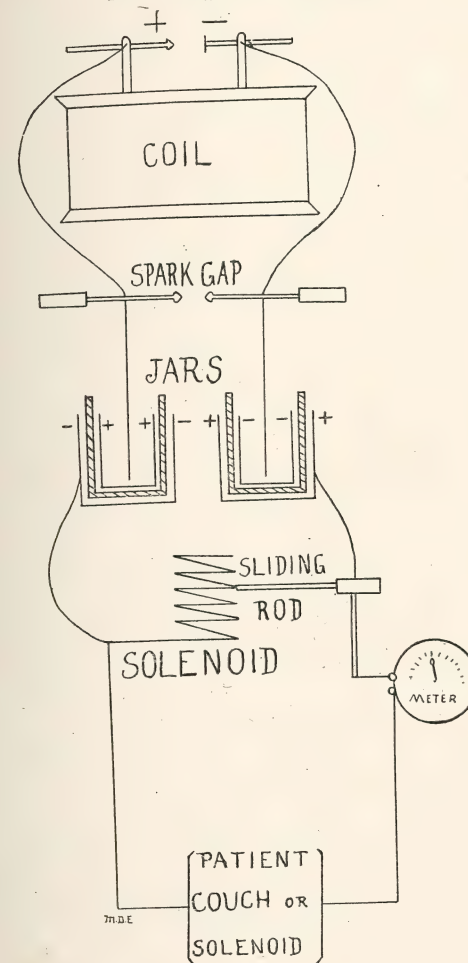
Fig. 13—Diagram of D'Arsonval Type.
