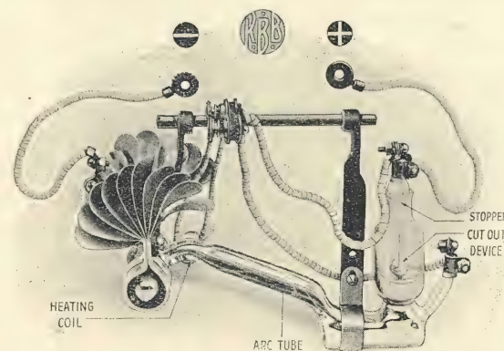
FIG. 6.—K.B.B. BURNER: 220-VOLT TYPE.
