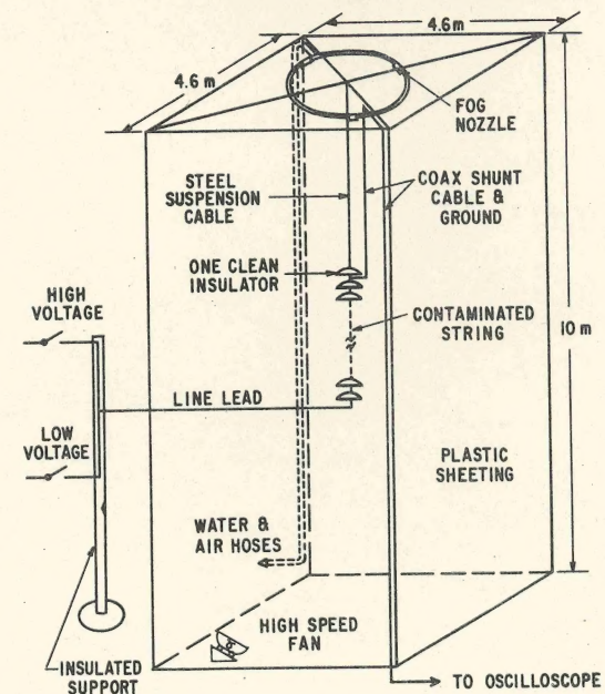
Fig. 2. Fog Chamber Arrangement.
