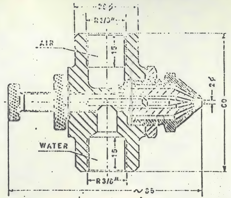
FIG. 5 LECHLER NOZZLE TYP Dr 112
