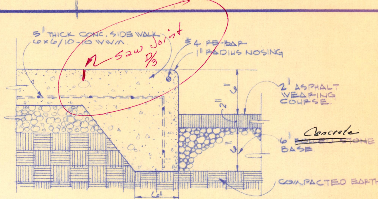
CUP-P DETAIL SCALE: 1/2" = 1'-0"
