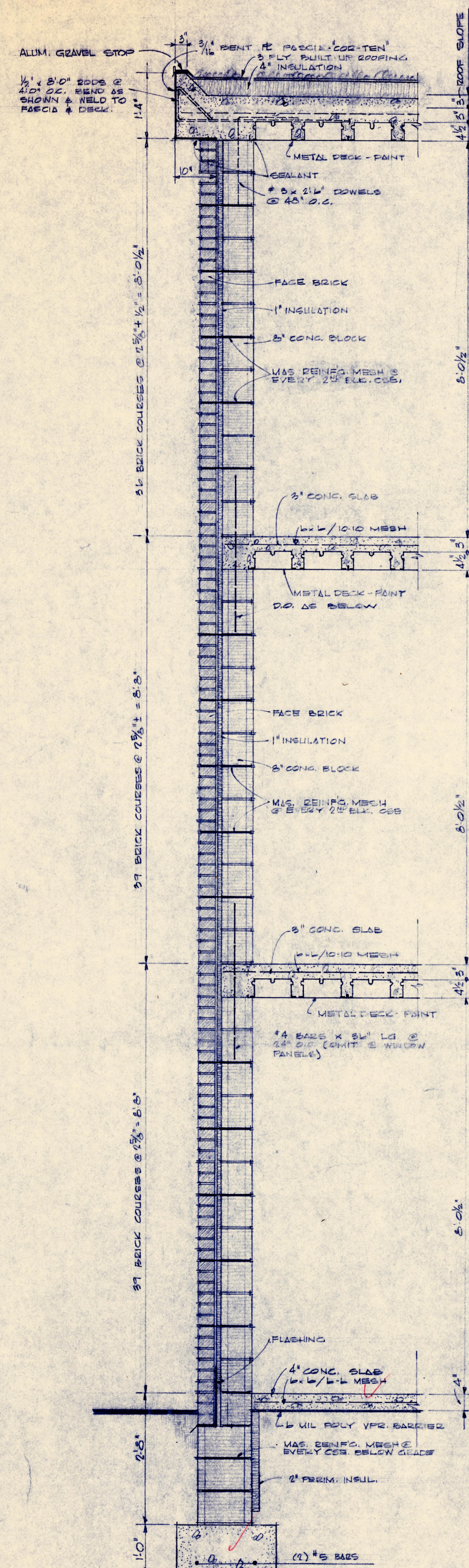
SECTION (A) SCALE: \frac{3}{4}'' = 1'-0''
