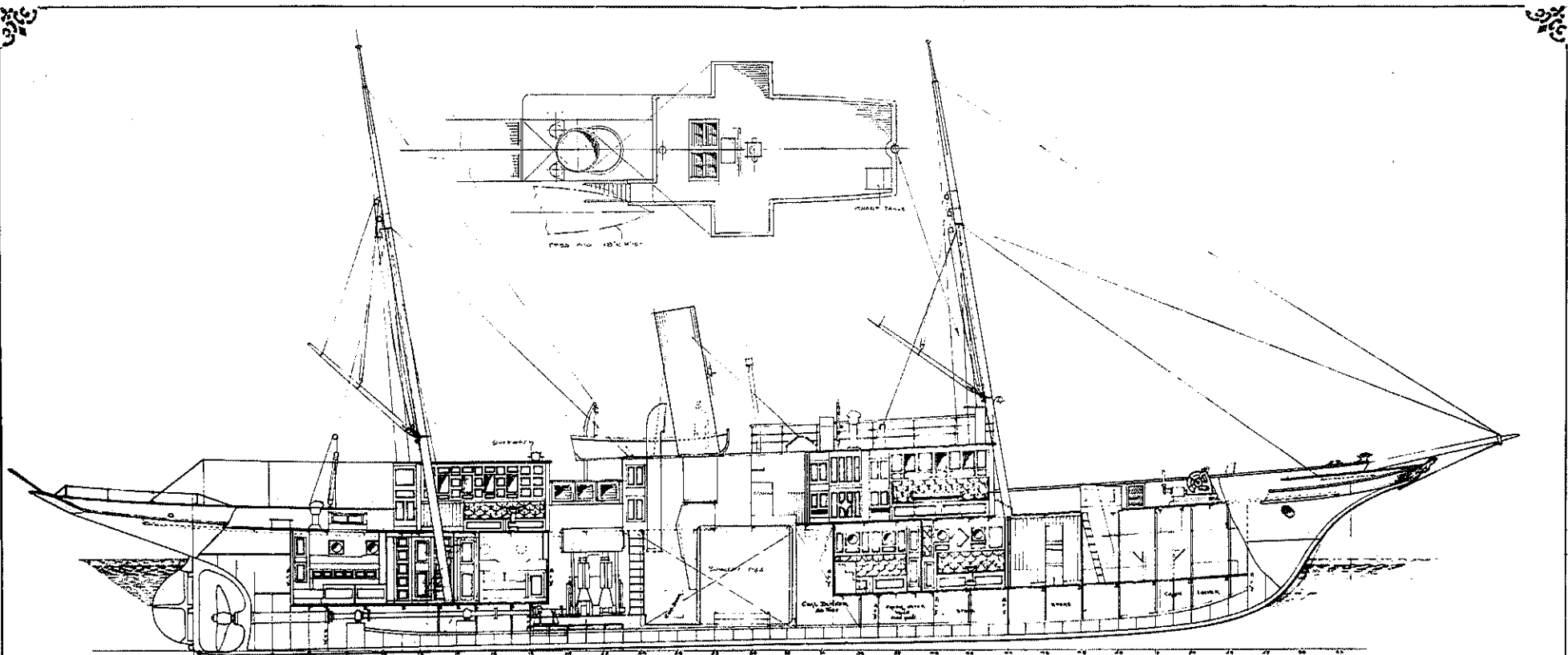
ELEVATION
