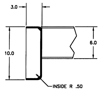
SECTION 96-A SCALE: 3"=1'-0
