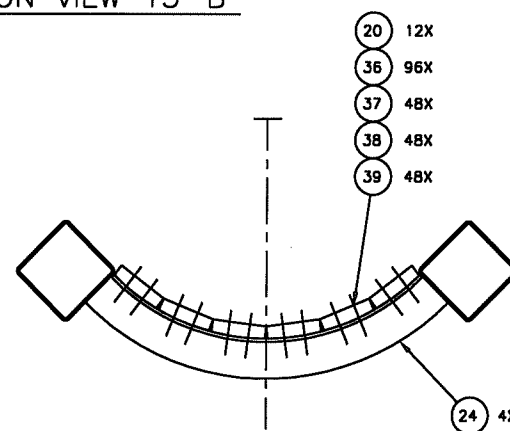
PLAN VIEW 12-A
