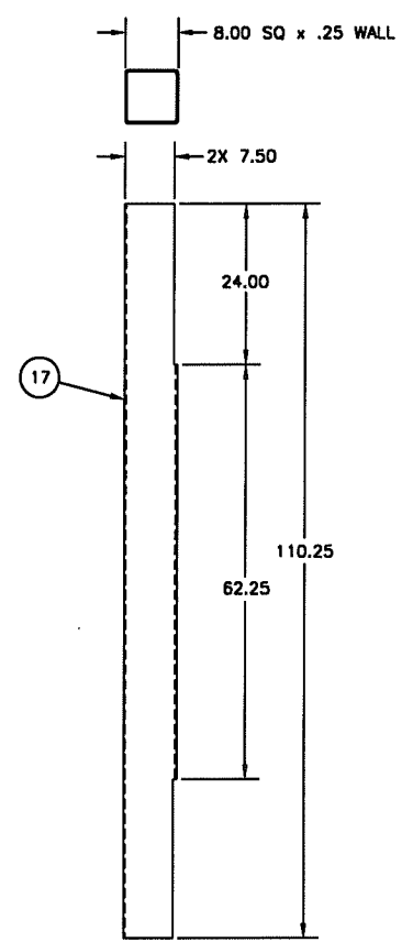
DETAIL 79-D SCALE: 1"=1'-0"
