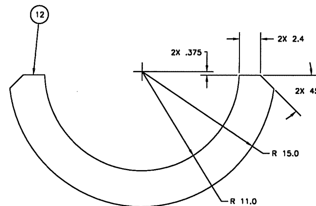
DETAIL 84-A
