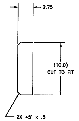
DETAIL 93-A SCALE: 3"=1'-0 TYP GUSSET DETAIL .25 THK PLATE
