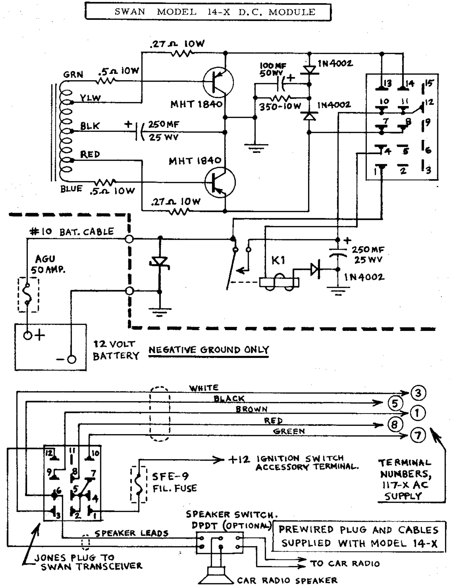
FIG. 8 MODEL 14-X D.C. MODULE
