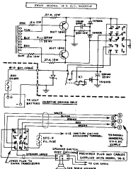
FIG. 8 MODEL 14-X D.C. MODULE
