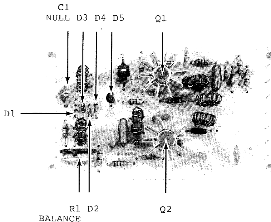
80452 RX MIXER
