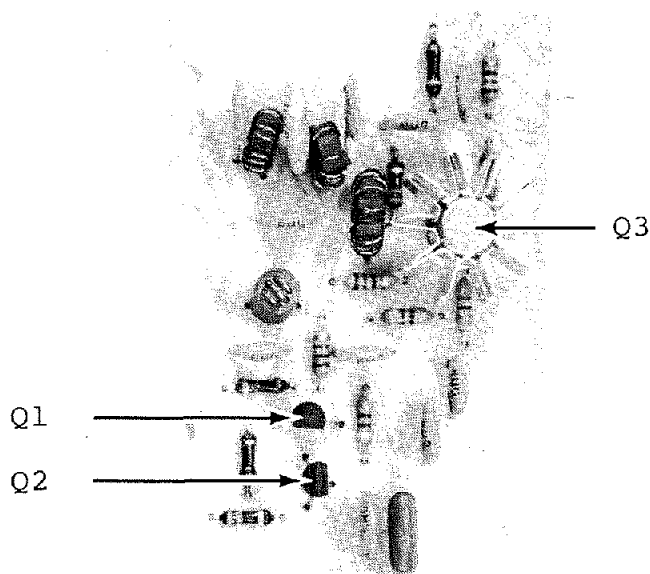
80454 VFO AMP
