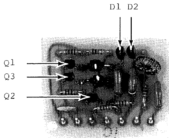
80445 RF ATTENUATOR
