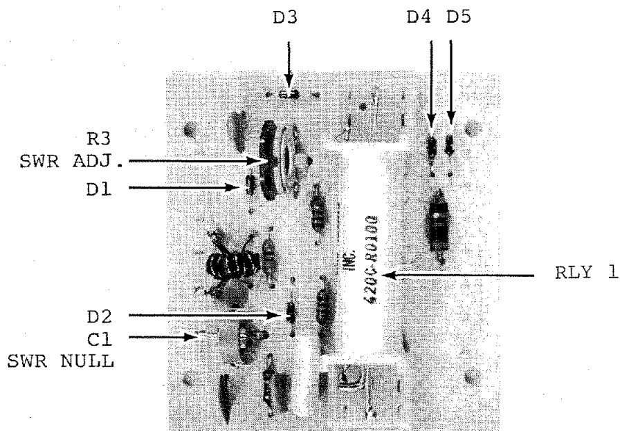
80450 SWR-TR
