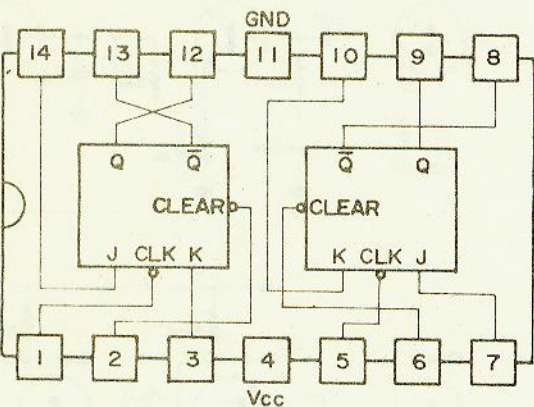
SN7473N
