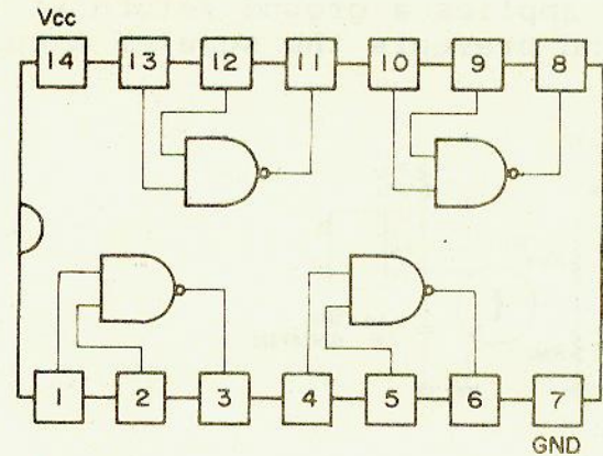
SN7472N
